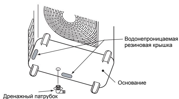
Дренажный патрубок
