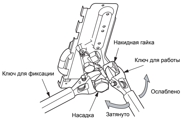
Клапан со стороны всасывания
